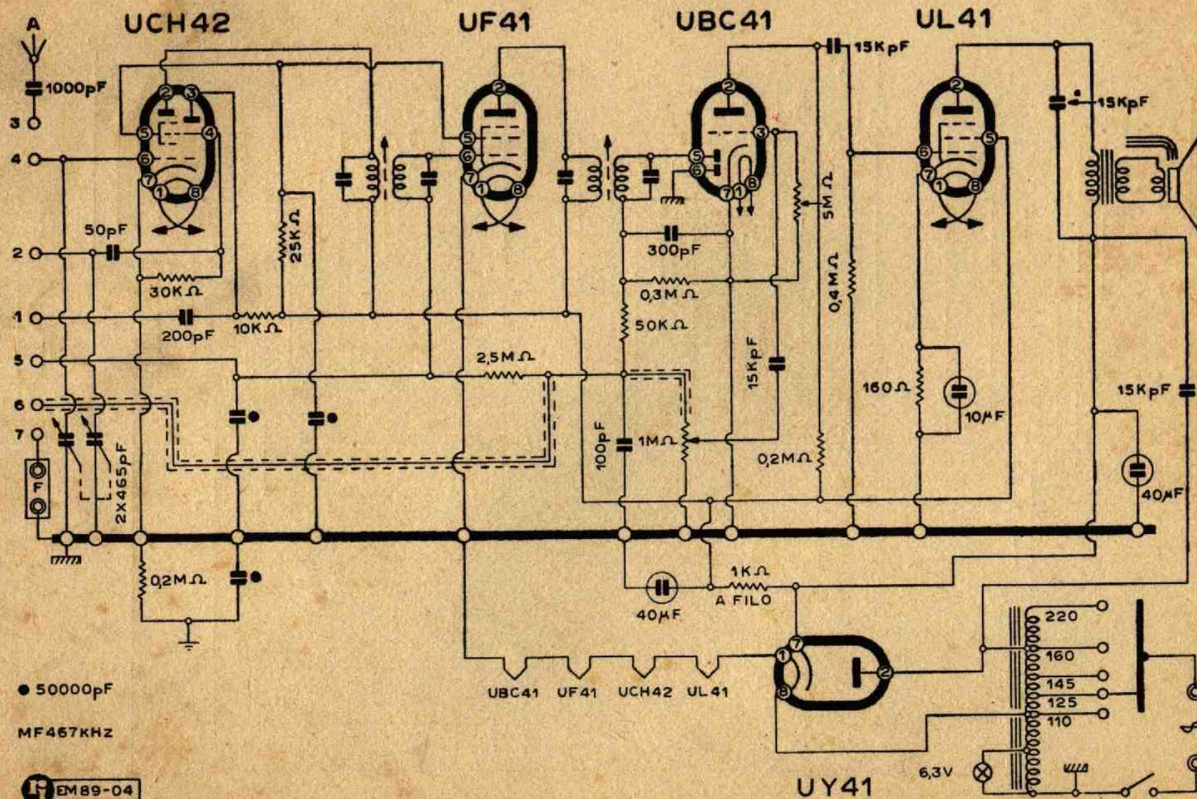
Lo schema elettrico del Mod. N0
